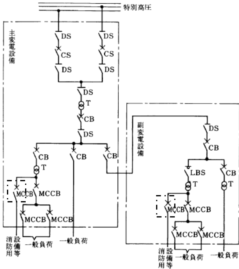
(イ) ループ方式配電例 (第37-2図参照) 第37-2図
