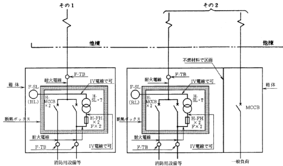
(イ) 計量器集合盤を用いた配電例 (第37-7図参照) 第37-7図
